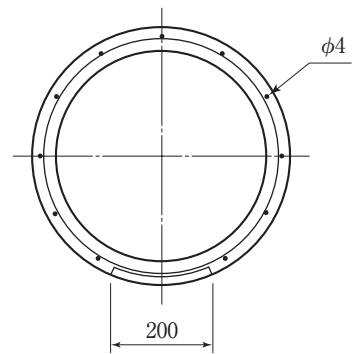
A-A'断面図
