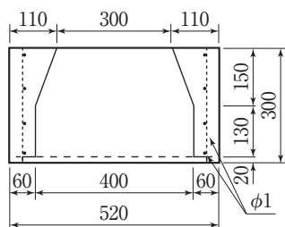
透水底塊
