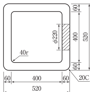
下部側塊
