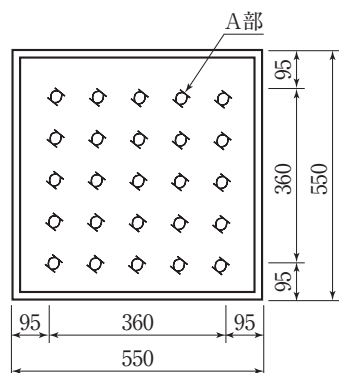
透水底塊
