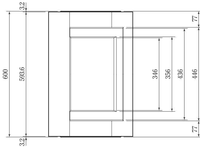
LU300(頭50)縁塊製品図
