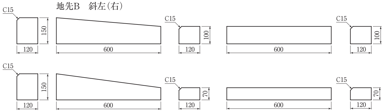
仕様寸法表(単位mm)
