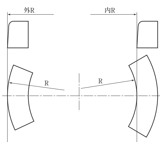
片面歩車道境界ブロック曲り
